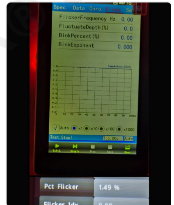
Flimmern: OHSP-350UVF 0 Hz, Modulationstiefe 0,0 %; UPrttek CV600 Flicker-Index 0,00.
