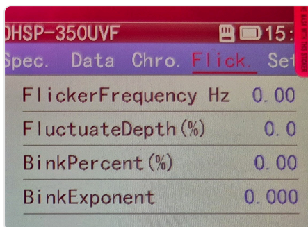
Migotanie: OHSP-350UVF przy 30 cm, głębokość wahań 0,0 %.
