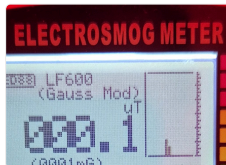
Cornet ED88 przy 30 cm: 0,1 \mu T.
