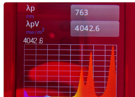
UPRtek CV600 przy 30 cm.
