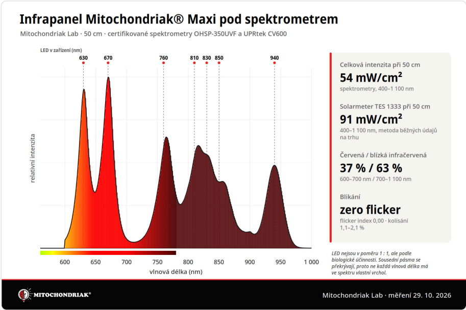
Spektrum při 50 cm, OHSP-350UVF, 560–1 000 nm, normalizované; pod 600 nm nula.
