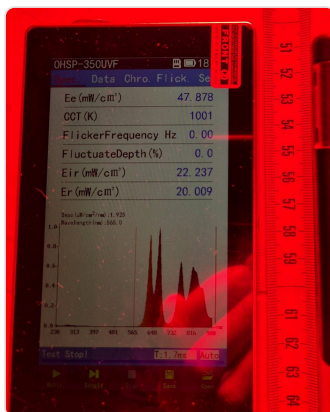
OHSP-350UVF bei 50 cm.
